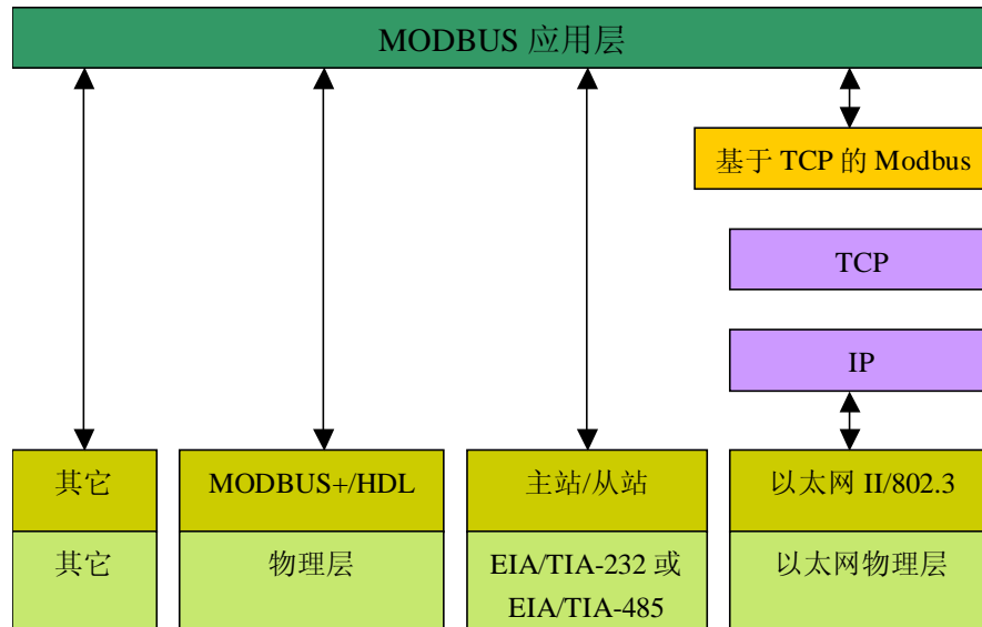
图 1：MODBUS 通信栈
