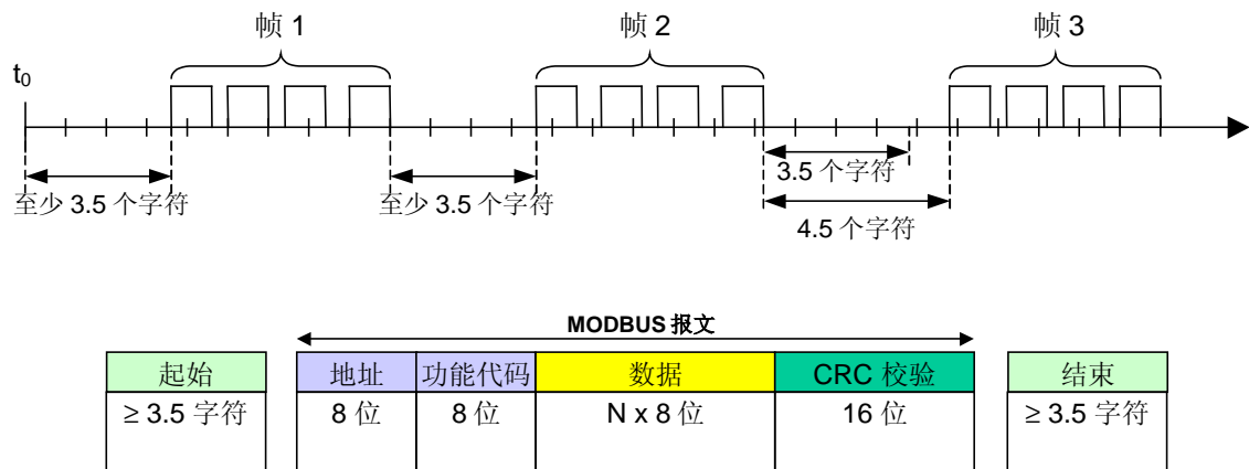
图 10: RTU 报文帧
