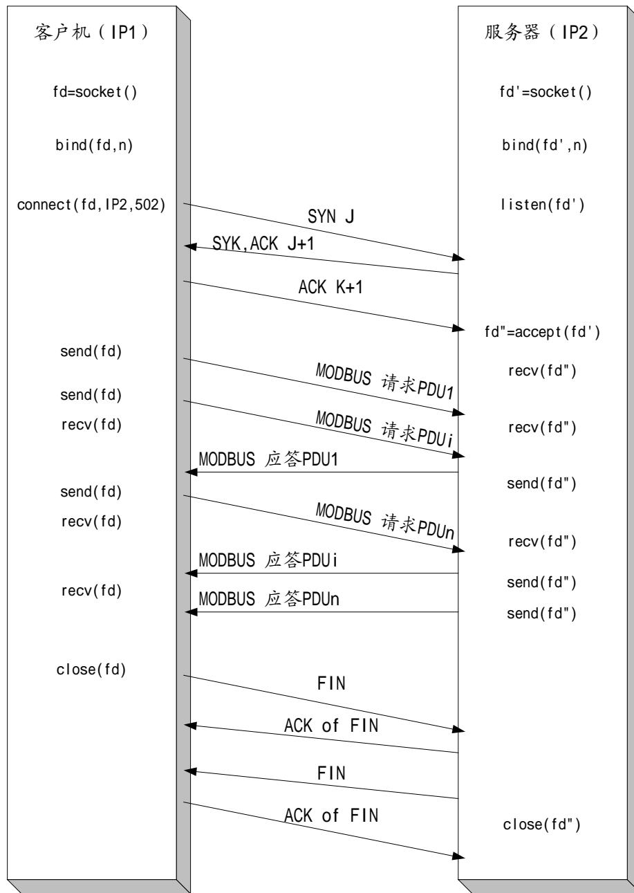
图9: MODBUS信息交换
