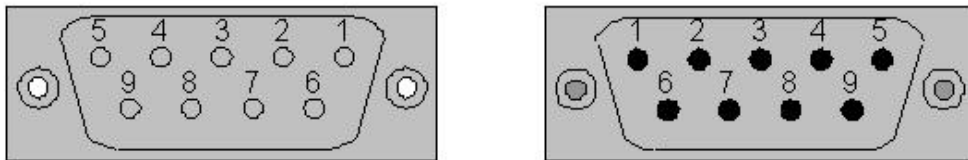
图 25： 9 引脚 D 型连接器
